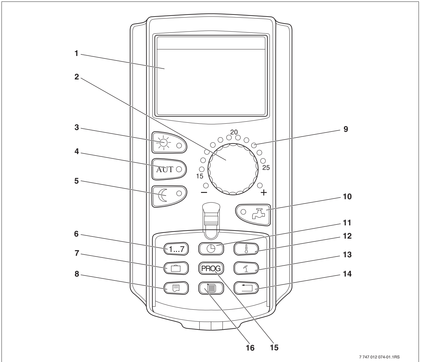
Рис.4 Пульт управления MEC2H
