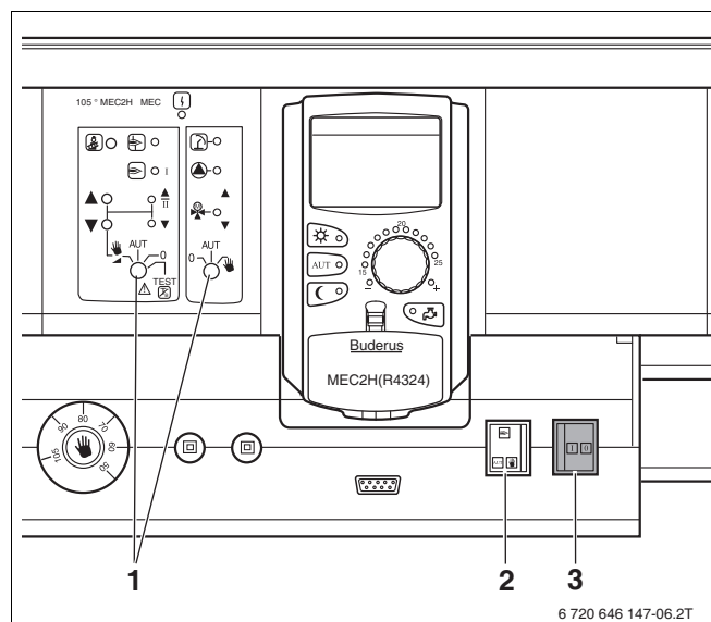
Рис.5 Пусковой выключатель
